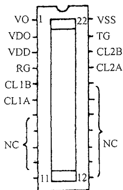
图 1-2-99 RL2048 引脚图
