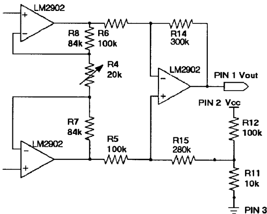
图3 差分放大电路
