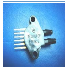
名称：MPX5050DP
