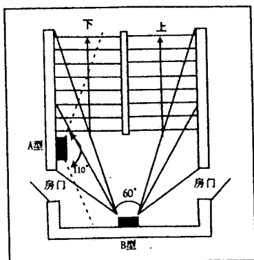
走廊安装示意图
