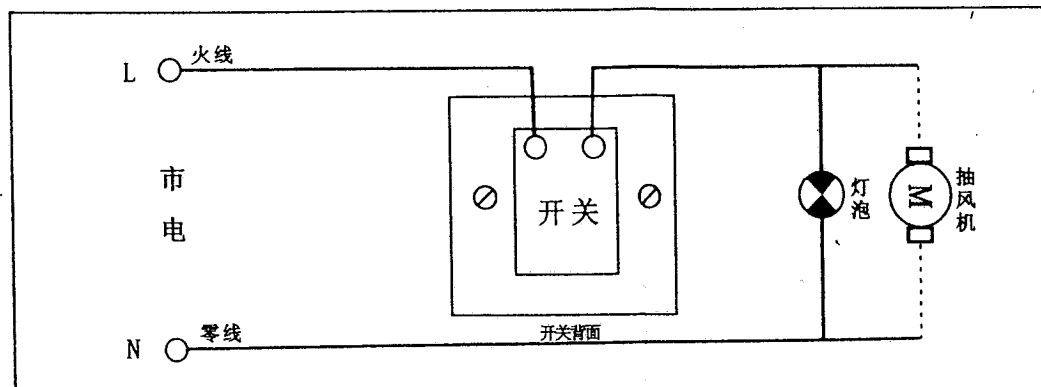
接线示意图
