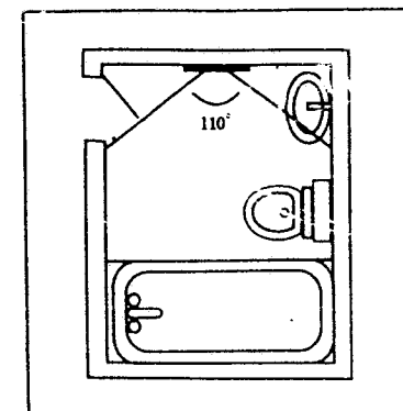
浴室安装示意图
