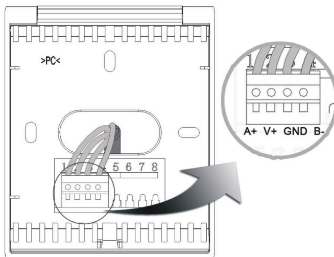
终端接线
