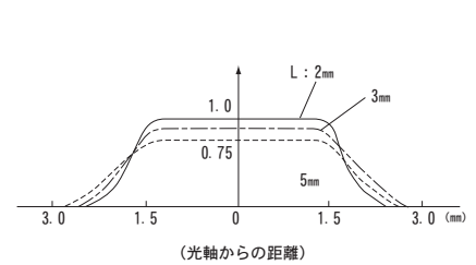
■相対光強度分布 ※2 RADIATION PATTERN
