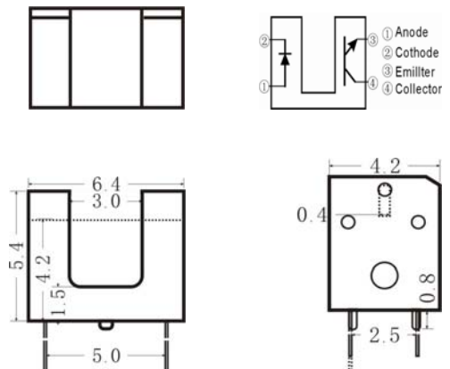
图.6 外形尺寸图 (单位: 毫米 ±0.1)
