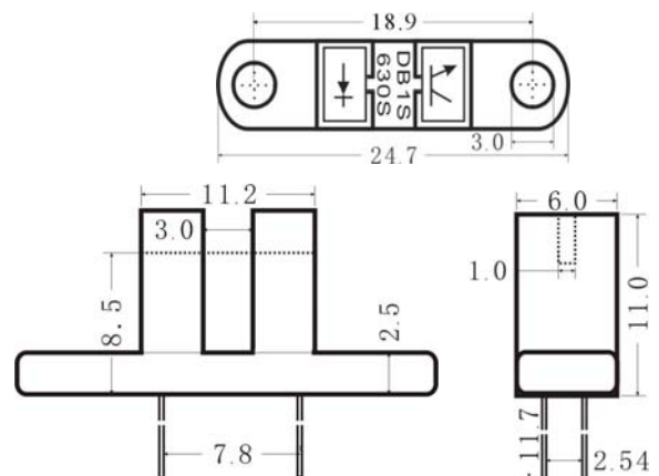
图.6 外形尺寸图 (单位: 毫米 ±0.1)
