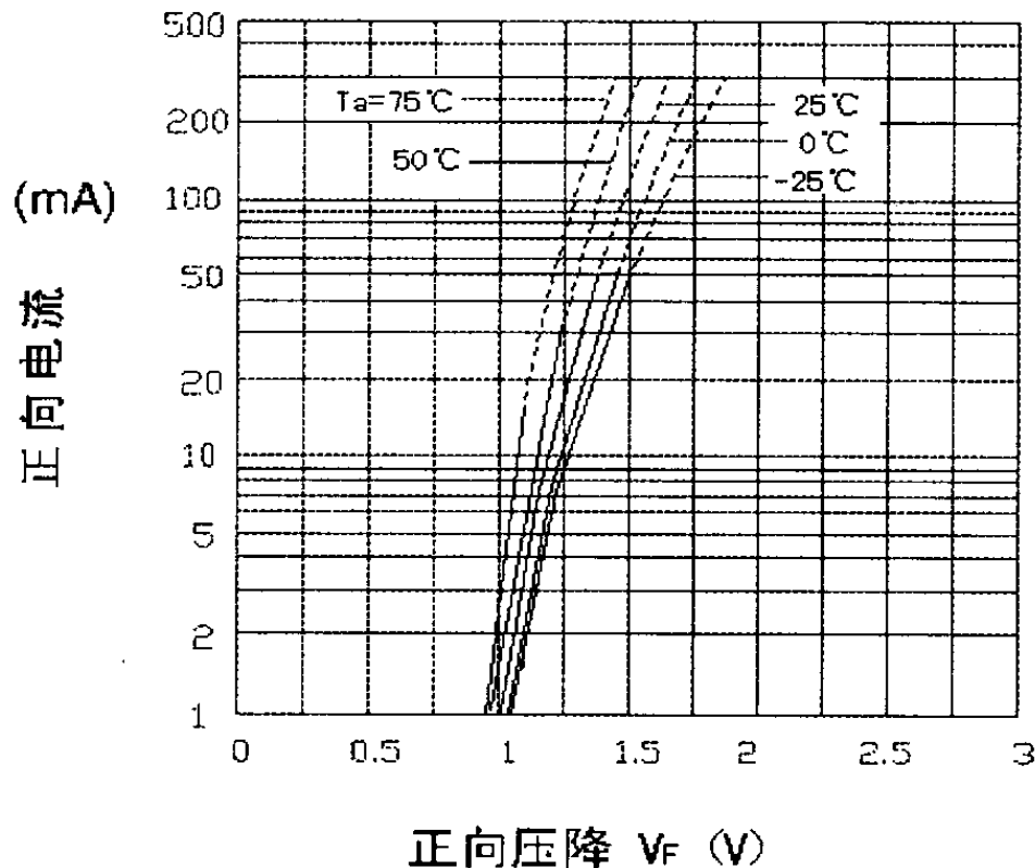
附图2. 正向电流与正向压降关系
