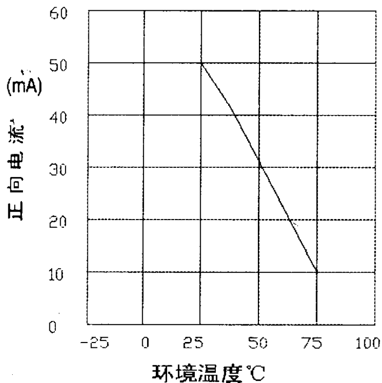
附图1. 正向电流与环境温度曲线图
