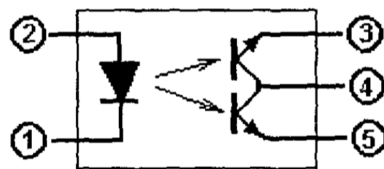
内部电路示意图
