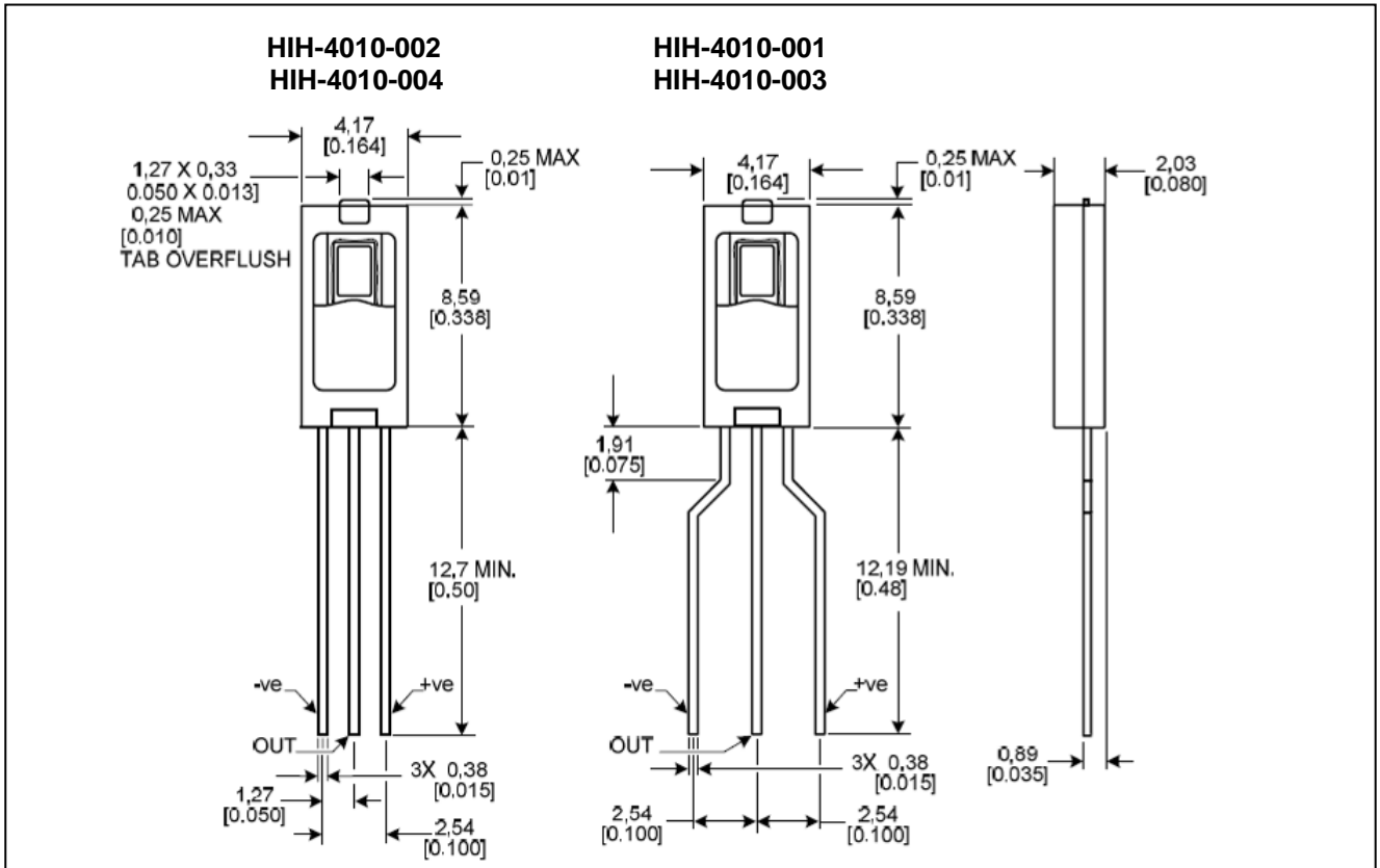
图 5. HIH-4010 系列安装尺寸 (仅供参考. mm[in])
