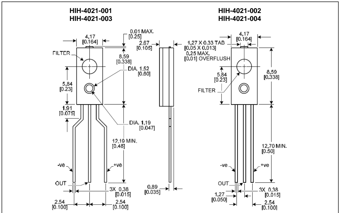
图 7. HIH-4021 系列安装尺寸 (仅供参考。mm[in])
