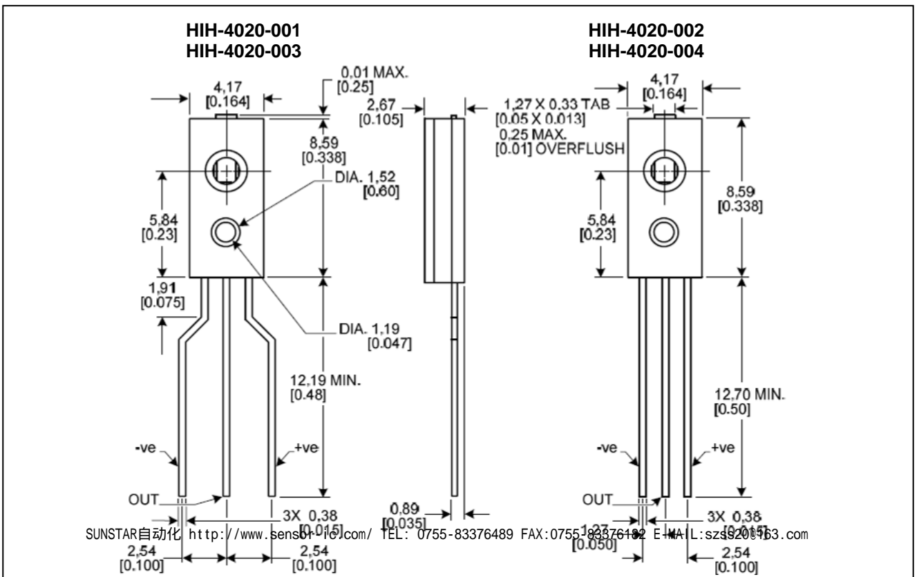
图 6. HIH-4020 系列安装尺寸 (仅供参考. mm[in])
