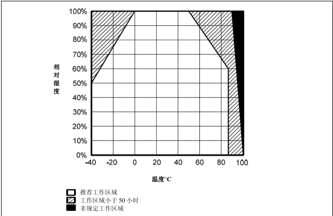
图 1. 工作环境 (型号 HIH-4010/4020 仅用于非冷凝环境)
