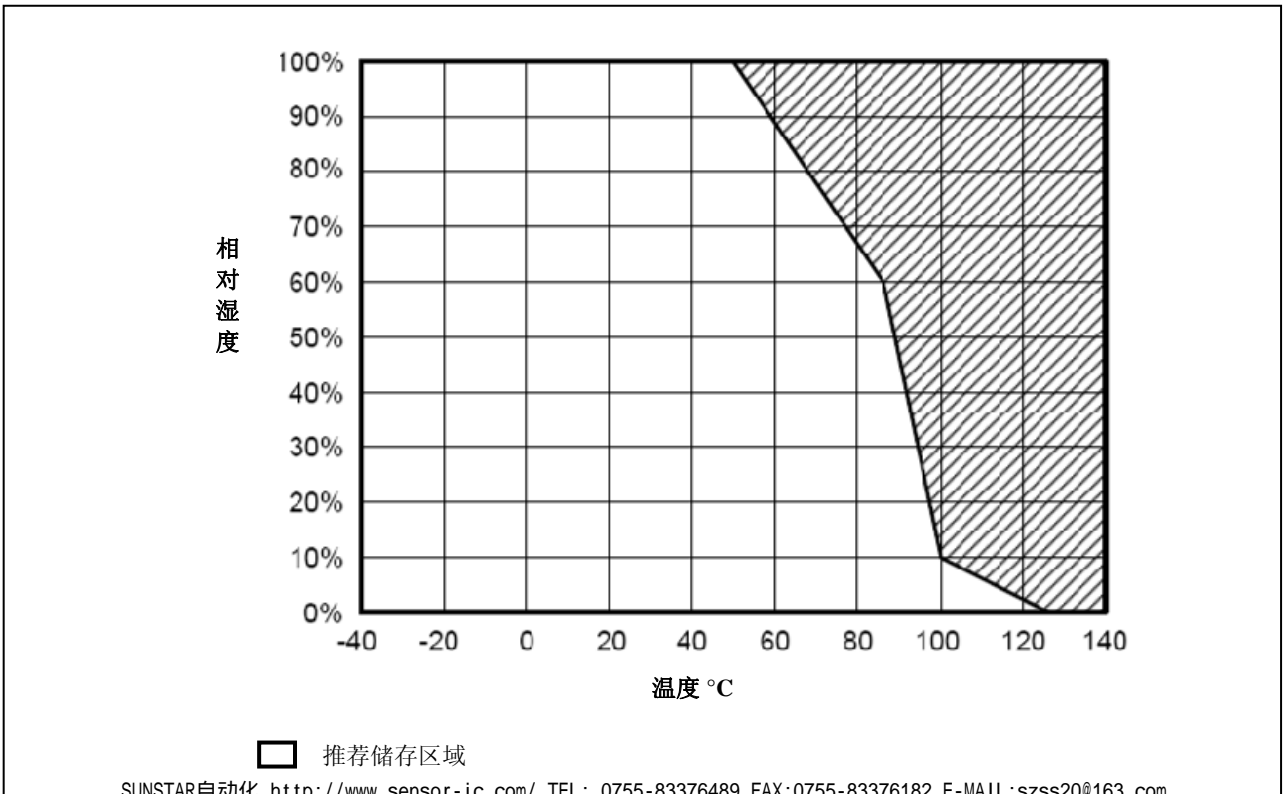
图 2. 储存环境 (型号 HIH-4010/4020 仅用于非冷凝环境)
