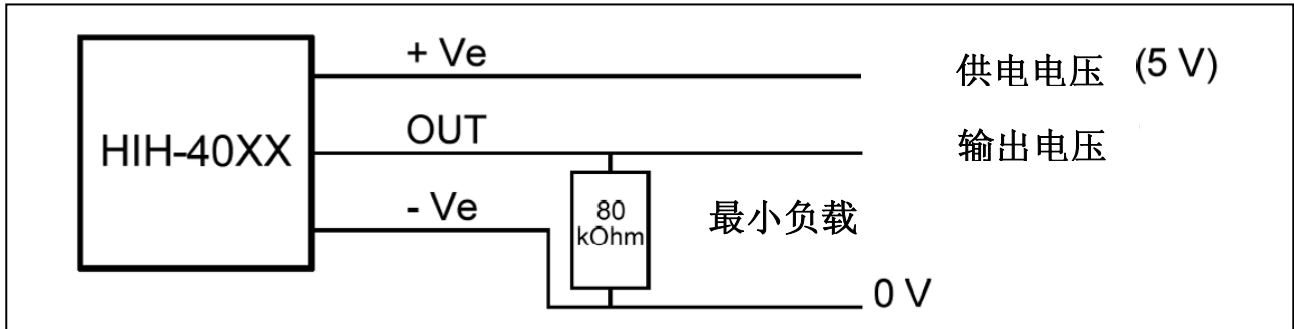
图 8. 典型应用电路
