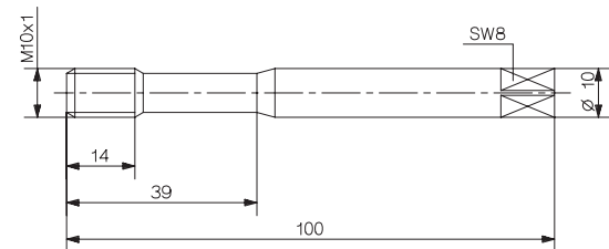
Fig. 13 : Taraud Type 1353
