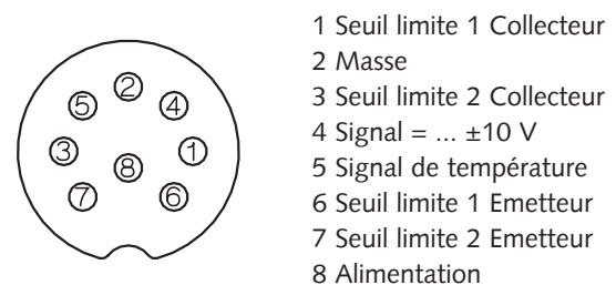
Fig. 9 : Connexions électriques de l'amplificateur
