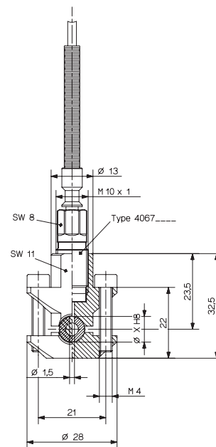
Fig. 16 : Adaptateur à bride Type 6533A1...
