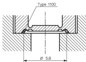
Fig. 5 : Etanchéité par joint métallique de Type 1100 Surface d'étanchéité trempée
