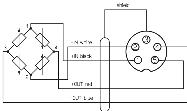
Fig. 8 : Affectation des broches du capteur
