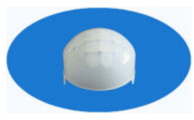
型号：7709-1B 焦距：7.6 角度：100° 距离：9m 尺寸：21 高度：12.72(16.8)
